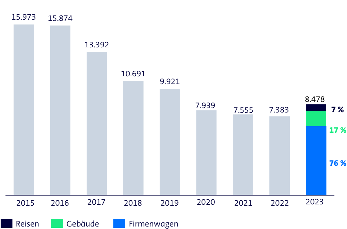
2015 – 2022: Entwicklung der CO 2 -Emissionen (t CO 2 ) und Hauptquellen
