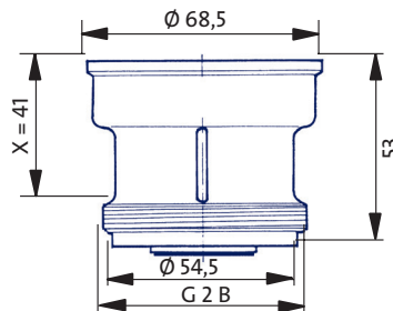
Abmessungen Verlängerung*
