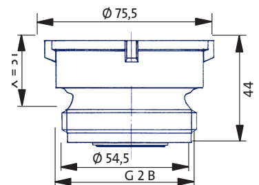
Abmessungen Fließrichtungsumwandler*
