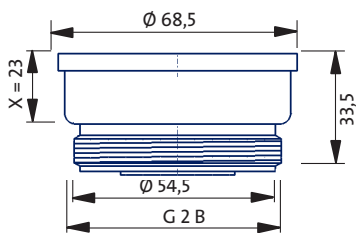
Abmessungen Verlängerung*
