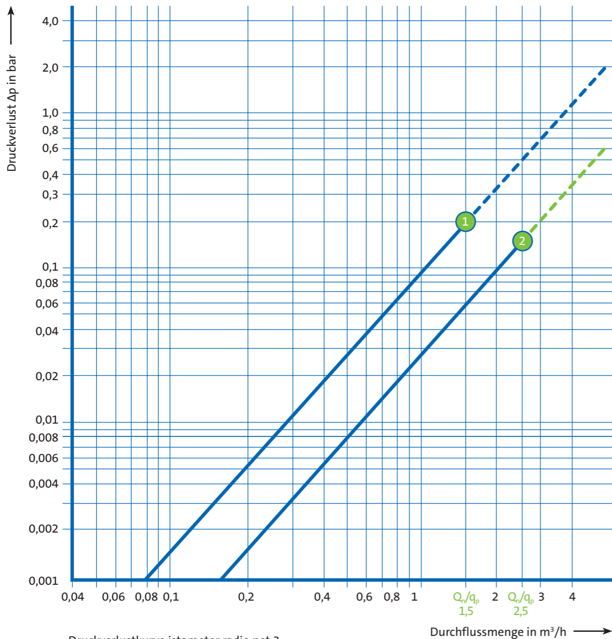
Druckverlustkurve istameter radio net 3 inkl. Einrohr-Anschlussstück (EAS)
