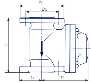
Maßbild 2 (Bauart WP)
