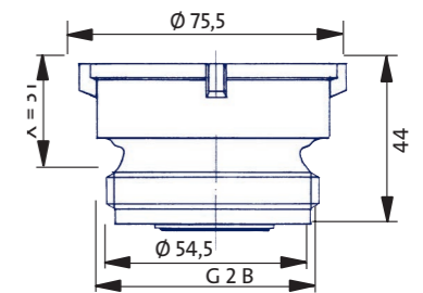
Abmessungen Fließrichtungsumwandler*
