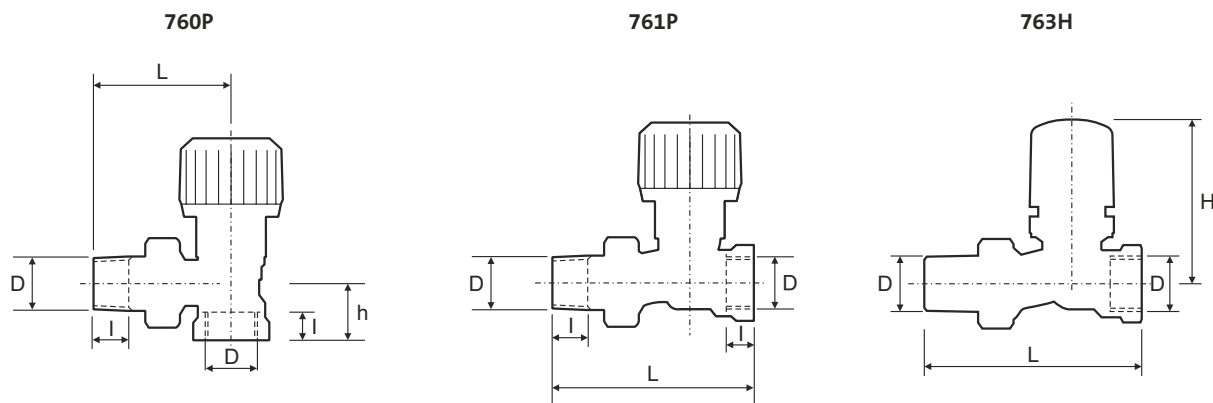
Габаритные и присоединительные размеры клапанов 760P, 761P, 763H
