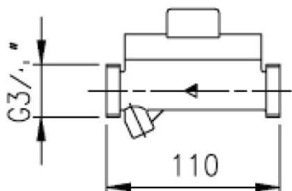
Versione filettata avente lunghezza 110 mm
