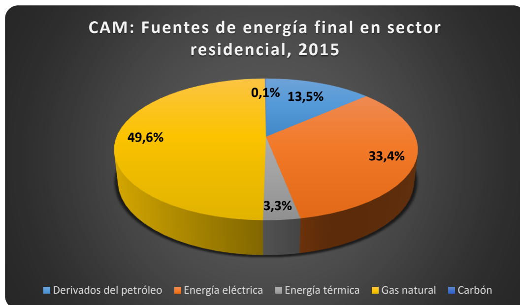
Figura 2.7. Fuentes de energía final en el sector residencial en la CAM, 2015.
