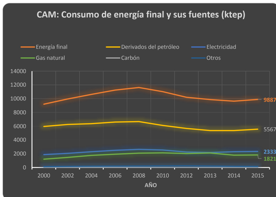
Figura 2.5. Consumo de energía final total y por fuentes. Comunidad de Madrid, 2000-2015.
