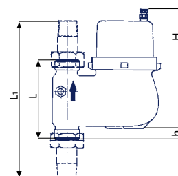
Plan de cote 2 (Exécution tube ascendant/descendant)
