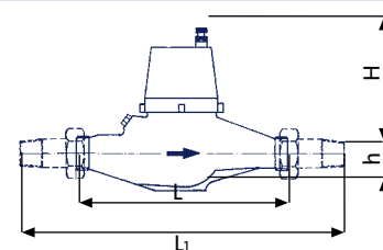
Plan de cote 2 (Exécution tube ascendant/descendant)
