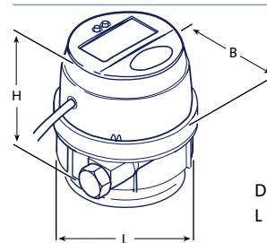
Plan de cote 1 (Exécution horizontale)
