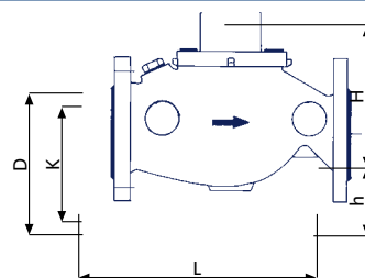
Plan de cote 3 (Exécution horizontale)
