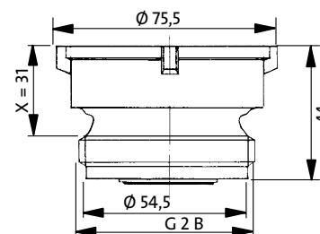
Dimension inverseur du sens d'écoulement*
