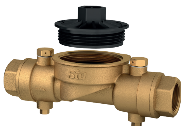
RMT avec deux robinets à boisseau sphérique intégrés (avec logement pour la sonde de température de retour)*
