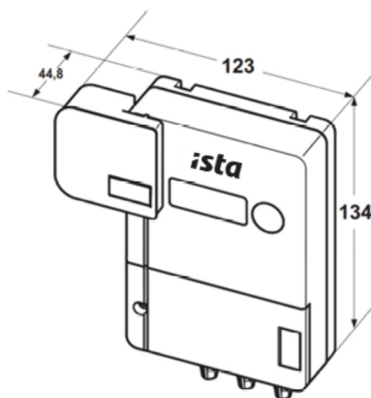
ista P4.0 z dodatkowym modulem
